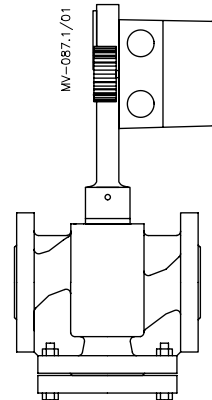
AMV 323, AMV 423, AMV 523 VL2/VL3 DN 15 - 100 mm
