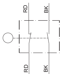
I простой выключатель
